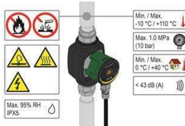
Figura 1: Líquidos bombeados, avisos e condições de funcionamento
